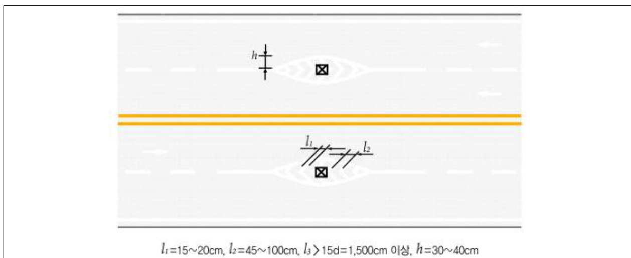
[그림 1] 안전지대 표시 설치 예시도
